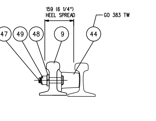
HEEL BLOCK ASSEMBLY
