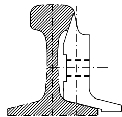
VIEW AT POINT END N.T.S.
