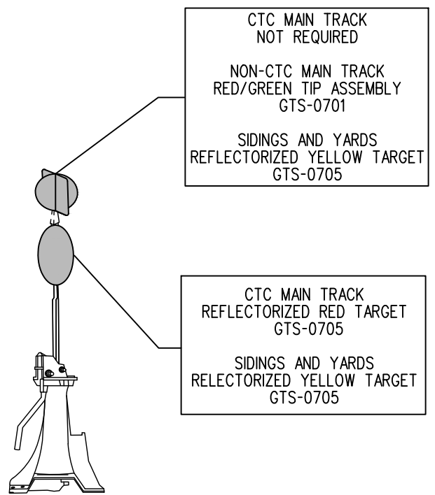
31 B SWITCH STAND
