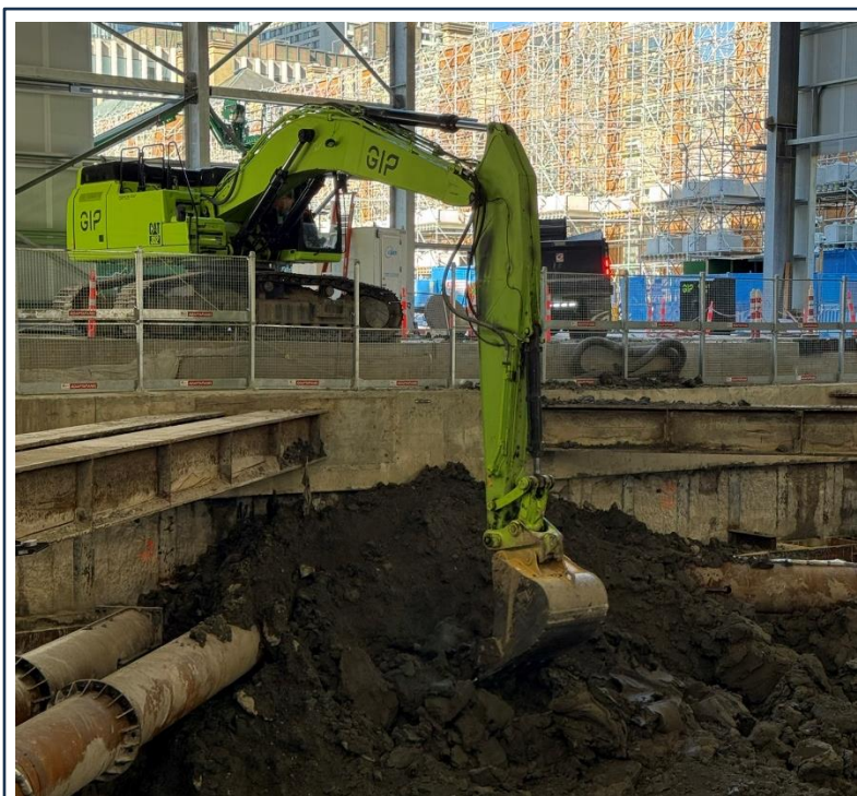
Excavation de sol meuble à l'extrémité nord du puits nord
