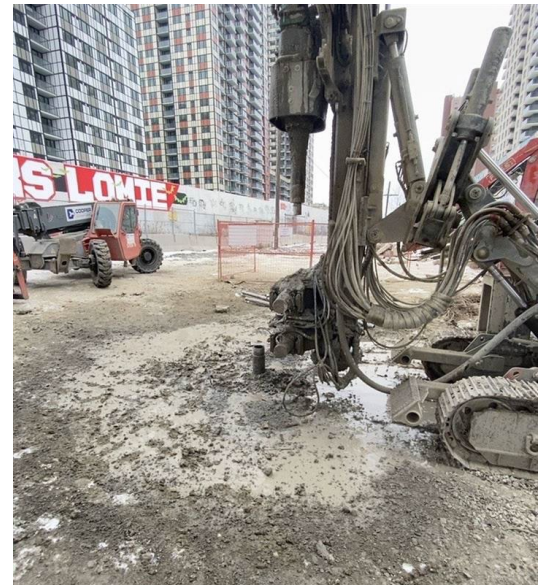
N° 5 Foreuse hydraulique utilisée dans le corridor ferroviaire
