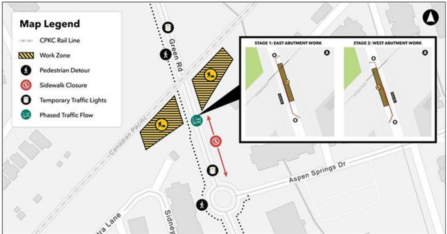
Figure 1 : Carte montrant la zone de travail et le plan de gestion du trafic associé sur le chemin Green. Non à l'échelle.
