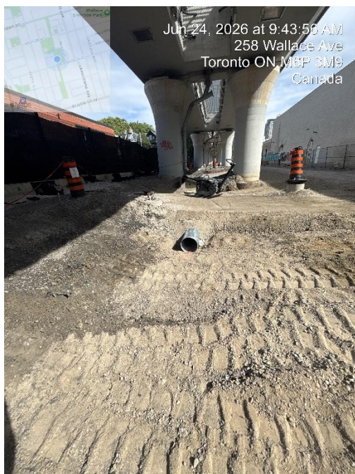
Installation de ponceau de drainage entre sur Wallace et Antler
