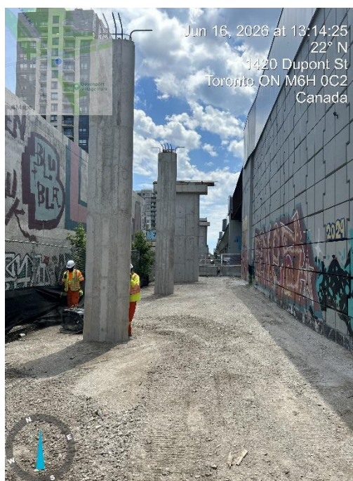
Terminé 4 sur 7 des piles de la passerelle piétonnière au nord
